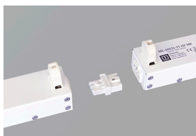
Vidarekoppling HF
