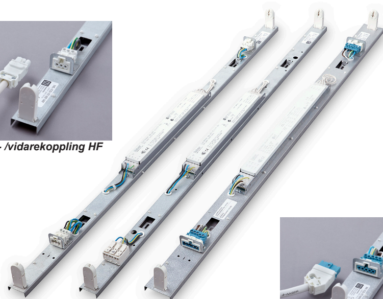
ML-T21-T5 HF ML-T21-T5 HF MF ML-T21-T5 HFD MF
